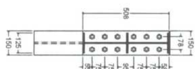
POT B-B 1:15
