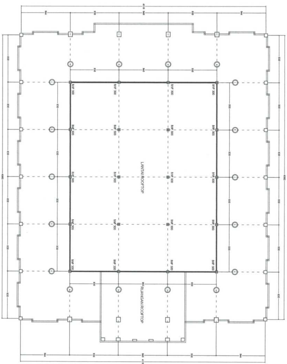
RENC. KOLOM ROOFTOP Skala 1 : 225
